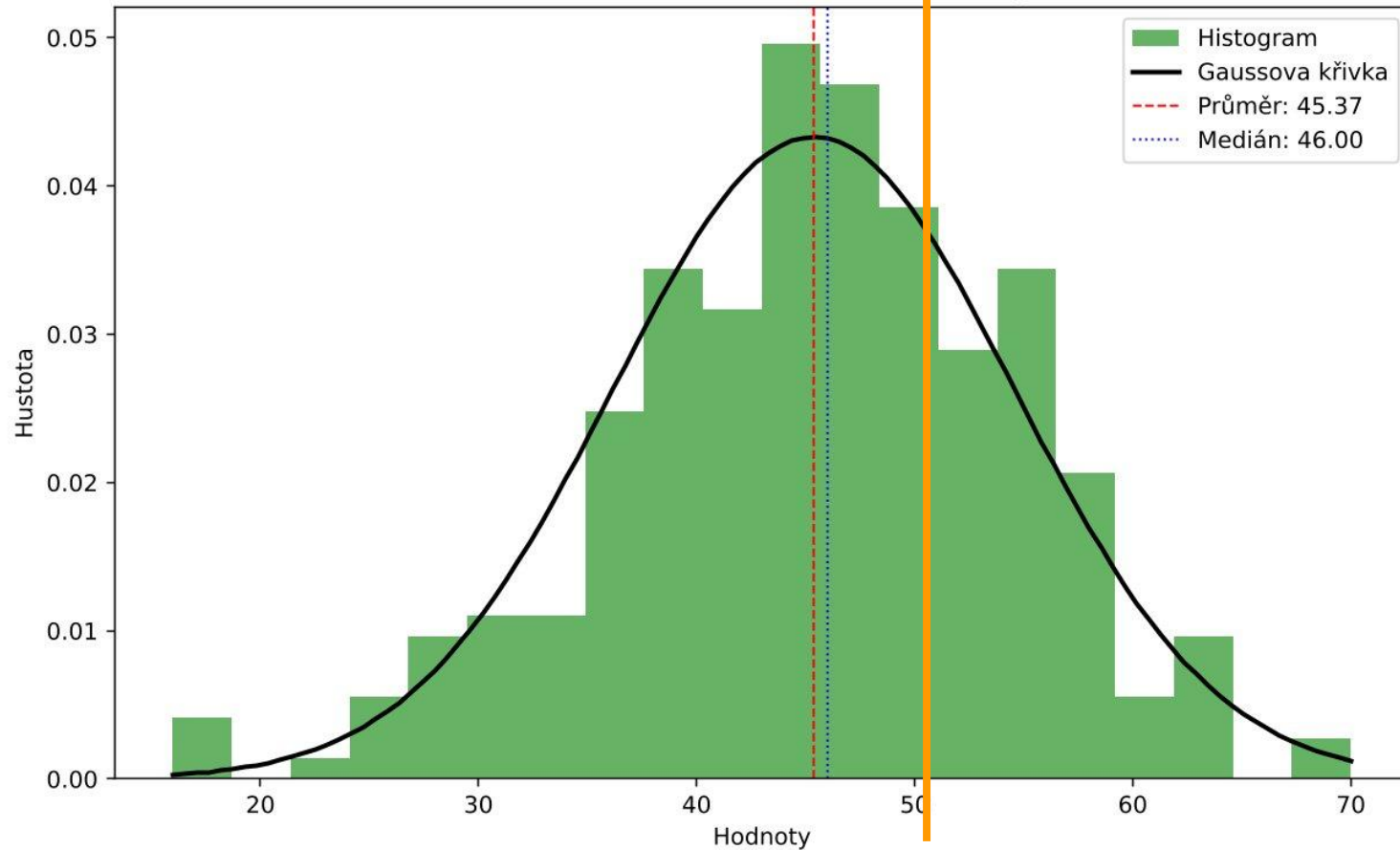
Normální rozložení (Gaussova křivka) s histogramem
